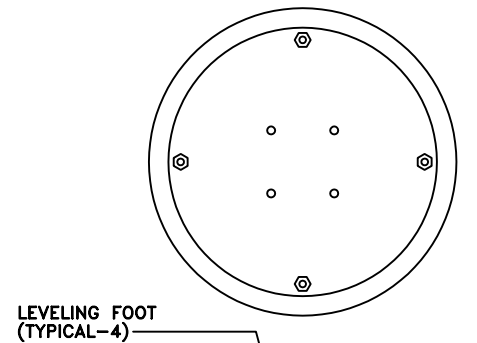
2814-OT-P (PEDESTAL MOUNT) SCALE: 3/4"=1'-0"
